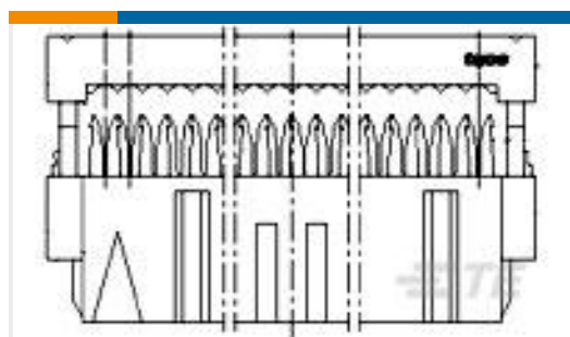
TE 产品编号1-215882-6 16 WAY GREY MK II RECP
