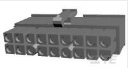
TE 产品编号770584-1 18P MINI UMNL PLUG HSG
