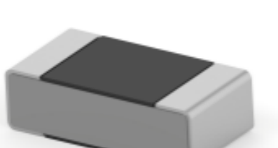
TE 产品编号4-1879132-0 RN 0402 23K2 0.1% 10PPM 1K RL
