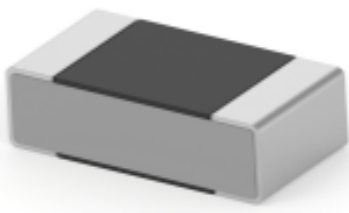
TE 产品编号7-2176269-0 RU 0603 15K 0.01% 2PPM 1K RL
