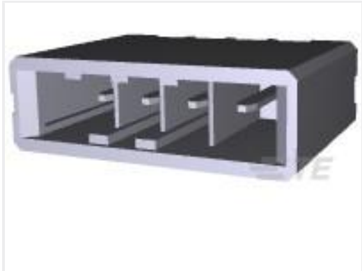
TE 产品编号1-917338-2 DYNAMIC 3200 VERTI. HDR ASY 4P
