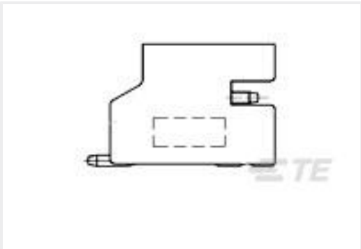
TE 产品编号1-1775469-4 HPI CONN., 2.0MM, R/A, SMT, 14P, 80U"
