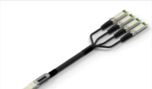
TE 产品编号4-2334878-4 QSFP TO [4]SFP 56GIG 26AWG 2 METER
