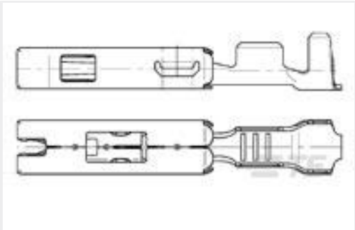
TE 产品编号929027-2 1.5MM SFC
