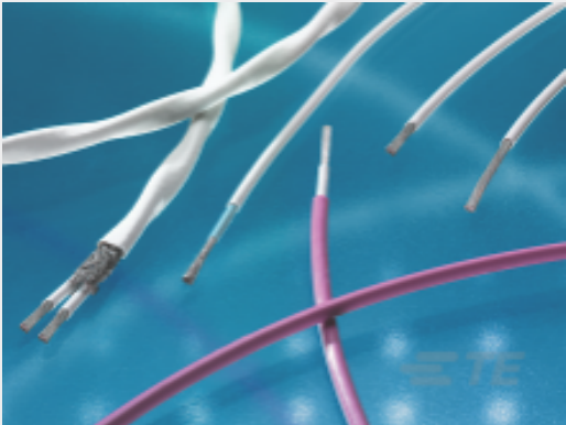
TE 产品编号CAT-55A-TC-3T24 通用 3 芯 TP 电缆，TC，24 AWG
