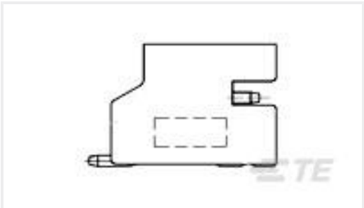
TE 产品编号1-1775469-4 HPI CONN., 2.0MM, R/A, SMT, 14P, 80U"
