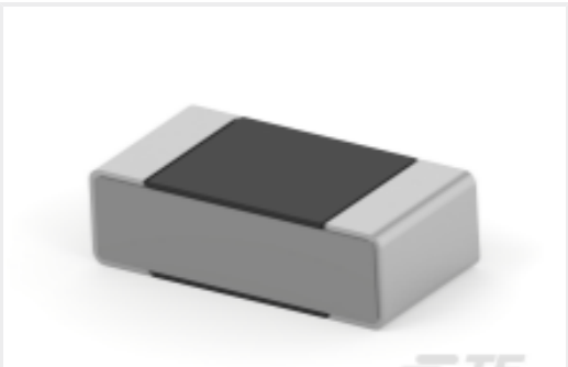
TE 产品编号4-1879132-0 RN 0402 23K2 0.1% 10PPM 1K RL
