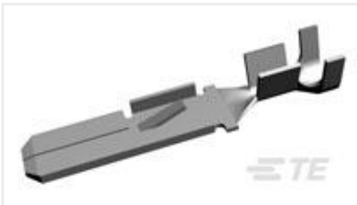
TE 产品编号153301-2 5.16 TAB
