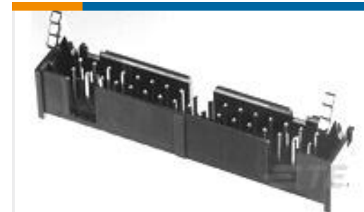
TE 产品编号3-1761606-1 IDC LOW PRO HDR 34P VERT LG LA PIN
