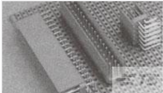
TE 产品编号281743-4 HEADER HE13 RA 2X4 P
