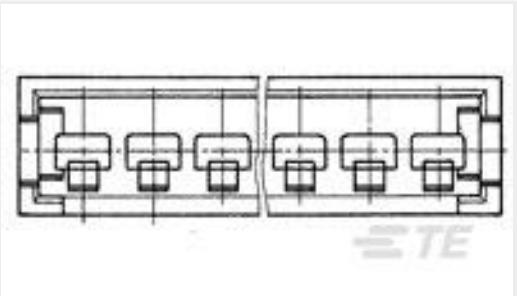
TE 产品编号 280635 AMPMODU II COSI PIN HSG, SGL ROW, 15 POS
