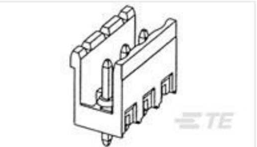
TE 产品编号282825-3 TERMI-BLOK HEADER,ASSY90 3P.5,
