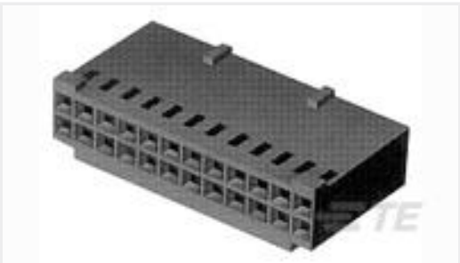
TE 产品编号 280369 AMPMODU II REC. HSG, DUAL ROW, 44 POS.
