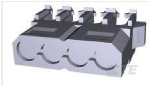
TE 产品编号770156-2 4P CMNL IDC PLUG 22AWG RED V2 AU
