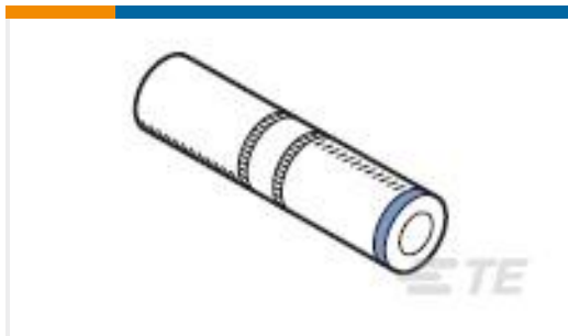
TE 产品编号 277159-1 SPLICE, COPALUM BUTT, 2 AL, 4 CU
