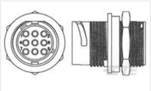
TE 产品编号 1445816-3 RECPT,11-9,FLNG MT,STD KEY
