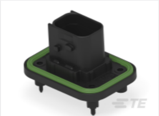
TE 产品编号1-2378182-1 8POS,TAB1.5X0.64,HDR ASSY, 180DEG,COD A
