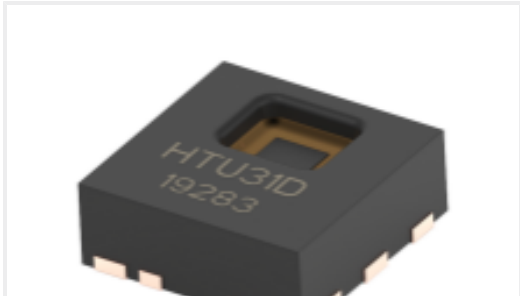
TE 产品编号10142048-30 HTU31V I.C 31V RH/T ANALOG R400
