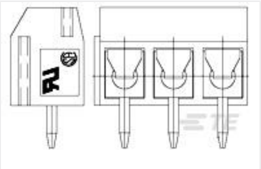
TE 产品编号1776244-2 2P TB ,90deg, VT, 5mm, Blue,w /interlock
