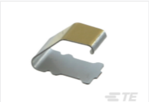
TE 产品编号1734300-1 SHIELD FINGER 3025-Z1-T
