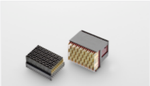
TE 产品编号2302789-2 VERTRECCASSY,CENTER,MULTIGIG RT3
