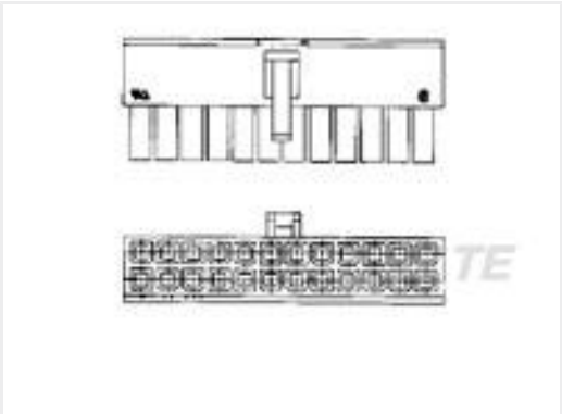
TE 产品编号2-794954-4 24P RCPT VAL-U-LOK V2
