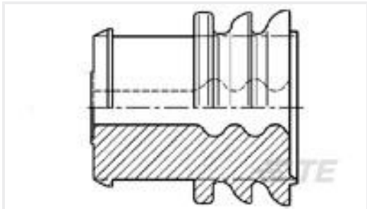
TE 产品编号963245-1 EINZELLEIT-DICHTUNG
