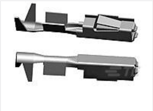
TE 产品编号5-963715-6 MQS0,63 Ag rec LL unseal. 0,5-0,75
