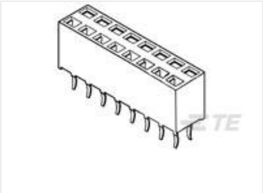
TE 产品编号215309-2 2X2P HV100 REC CON. TE, 8.5MM
