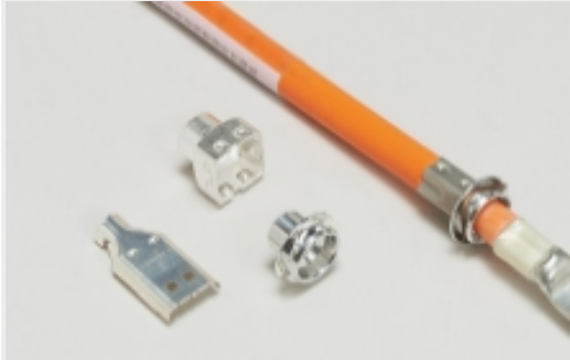
汽车连接器 EMC 屏蔽(4)
