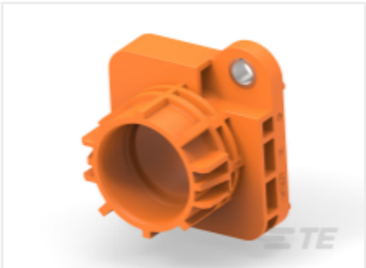
TE 产品编号 2-2443905-1 PROP,IPT-HD-1P-ASSY-50-95MM2- CODE-B
