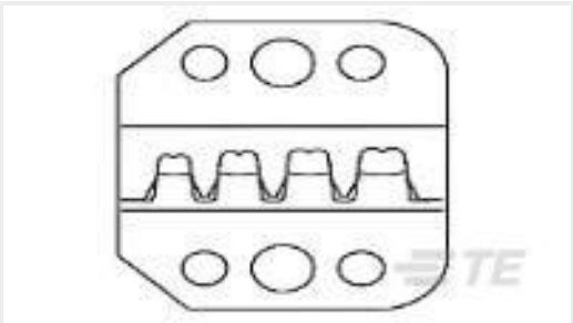
TE 产品编号90548-2 PROCRIMPER DIE ASSY UNIV MNL
