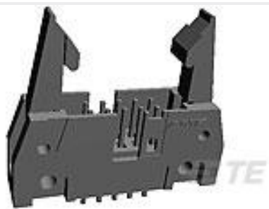
TE 产品编号1-5499922-2 A/L UNIV HDR 64P VERT LAT
