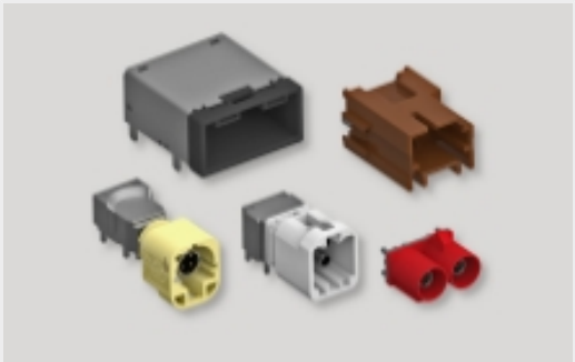
数据连接器接头(360)
