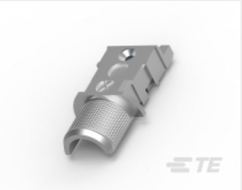
TE 产品编号1823954-1 FAKRA II, PLUG
