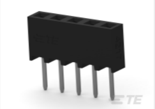
TE 产品编号 2314869-4 4P,2MM,BB,REC,SRVT,2.0,0.38AU,TB, W/CAP
