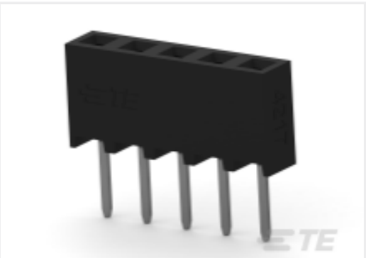
TE 产品编号 2307772-4 4P,2MM,B-B,REC,SRVT,3.2,0.38AU, TUBE
