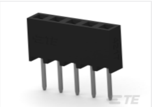
TE 产品编号 2307771-4 4P,2MM,BB,REC,SRVT,2.7,0.38AU,TR, W/CP
