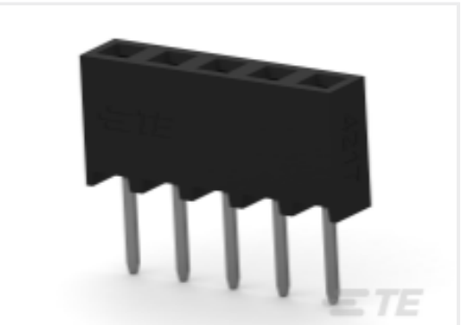
TE 产品编号 2314881-4 4P,2MM,BB,REC,SRVT,2.7,0.38AU,TB, W/CP
