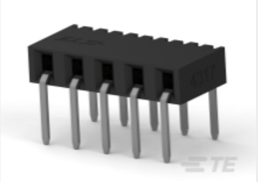
TE 产品编号 2307708-4 4P,2MM,B-B,REC,SRHZ,3.4,0.38AU, TUBE
