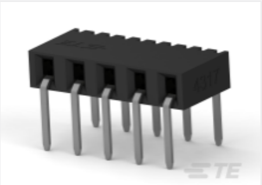
TE 产品编号 2307707-4 4P,2MM,B-B,REC,SRHZ,2.8,0.38AU,TB
