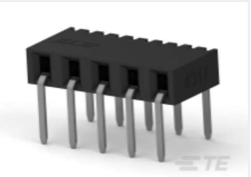
TE 产品编号 2314929-4 4P,2MM,B-B,REC,SRHZ,2.1,0.38AU,TB
