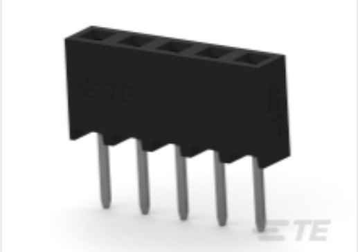
TE 产品编号 2314877-4 4P,2MM,B-B,REC,SRVT,2.7,0.38AU,TB
