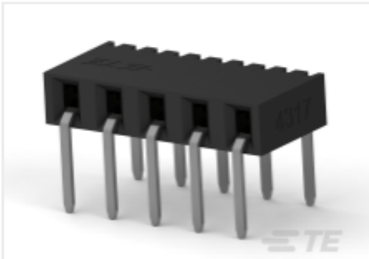
TE 产品编号 2307703-5 5P,2MM,B-B,REC,SRHZ,2.1,0.1AU,TR
