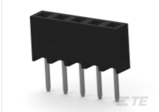
TE 产品编号 2314868-5 5P,2MM,BB,REC,SRVT,2.0,0.1AU,TB,W/CP
