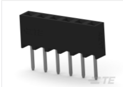
TE 产品编号 2314868-6 6P,2MM,BB,REC,SRVT,2.0,0.1AU,TB,W/CP
