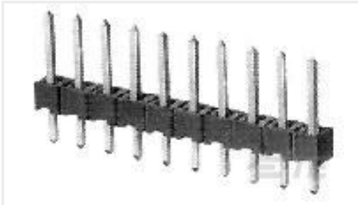
TE 产品编号826646-5 5P AMPMODU II STIFT LEI
