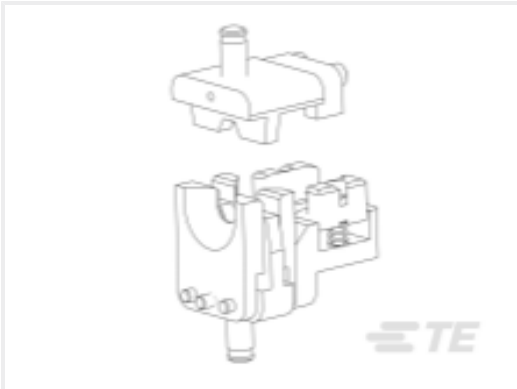
TE 产品编号2234130-1 DIE SET HVA280-2P/3P F
