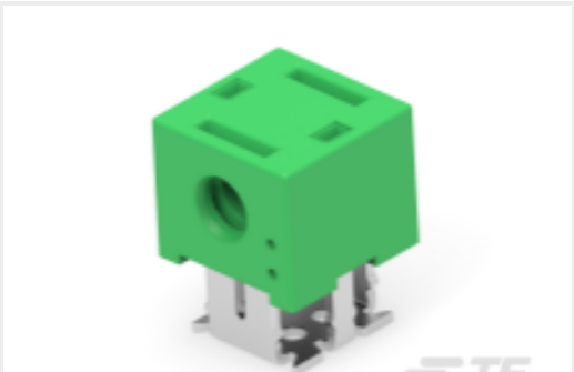
TE 产品编号474339-E IDCTERM 1 I2426 1,10 * 167 707 0007 J 2
