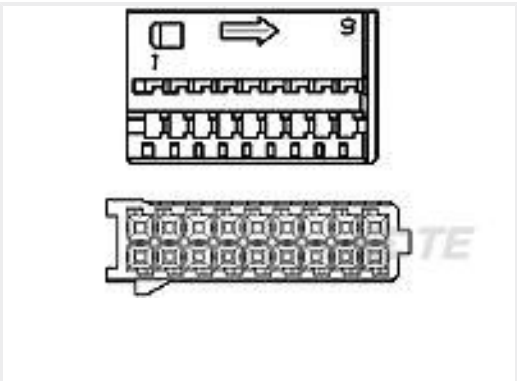
TE 产品编号1355348-1 18POS MQS REC
