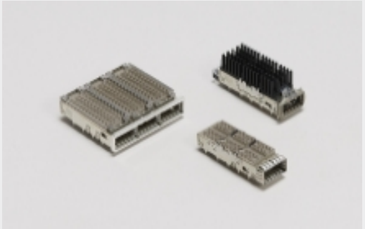
QSFP、QSFP+ 和 zQSFP+(401)
