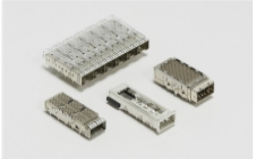
插拔式 IO 连接器和笼子(401)
