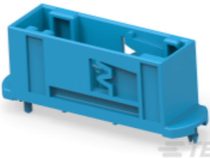
TE 产品编号2137614-2 32P MQS Header
