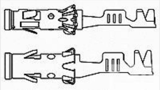
TE 产品编号929975-1 BU-KONTAKT 2,5MMMD
