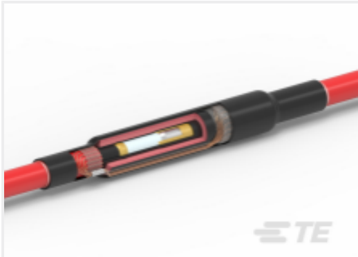
TE 产品编号CAT-MXSU-INL-1C 12-42 kV 热缩电缆接头
