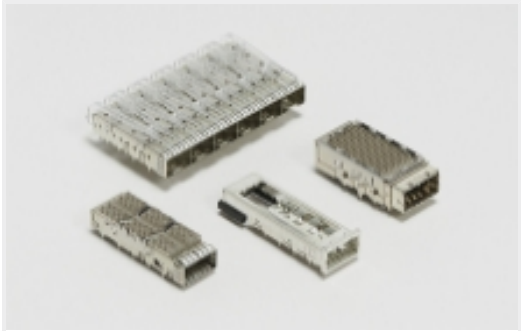
插拔式 IO 连接器和笼子(3)
