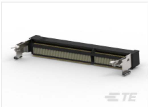
TE 产品编号 2-2013310-1 EMBOSS TAPE DDR3 204P 9.2H STD
