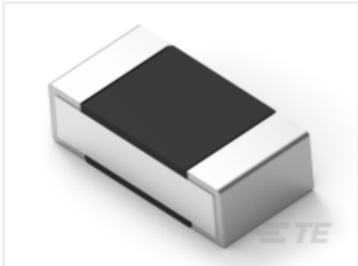
TE 产品编号2176309-7 RP 1E 0.1W 11R5 0.1% 25PPM 1K RL
