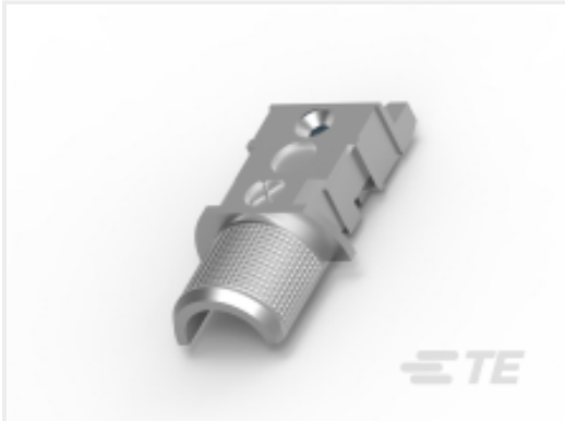
TE 产品编号1823954-1 FAKRA II, PLUG
