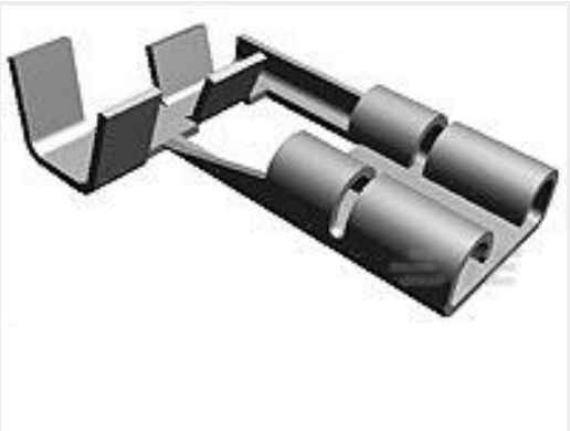
TE 产品编号100645-3 250 FASTON,FLAG,REC.,14-17AWG, PHBRZ
