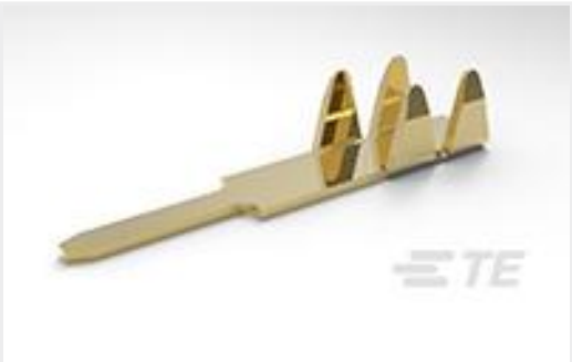
TE 产品编号1-88997-2 FFC S.TAB 100SN RL
